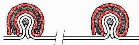
CP外周スチールガイド樹脂カバーの断面構造
